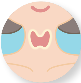
甲状腺
