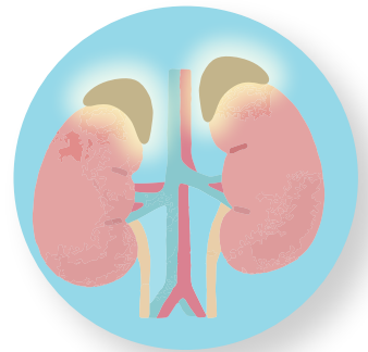
副腎
